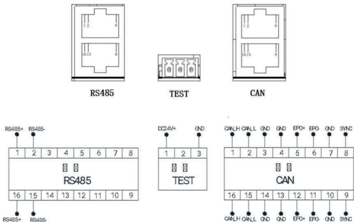
Rysunek 7. Wejścia sterownicze RJ45
