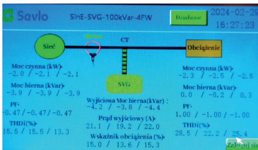
Rysunek 32. Ekran główny w trakcie działania
