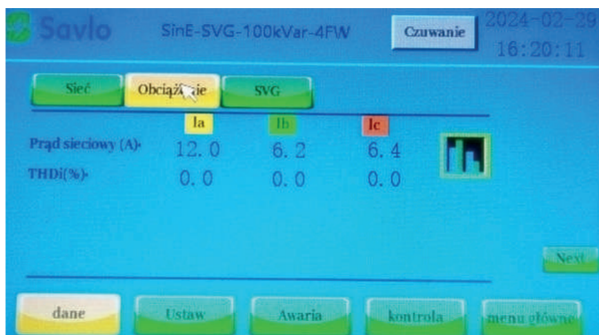
Rysunek 14. Ekran danych, strona odbioru, obciążenia
